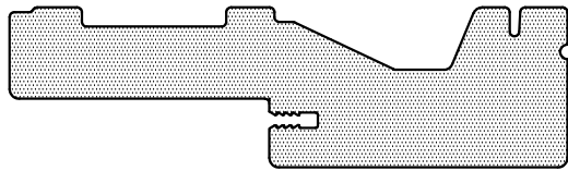
PVC JAMB
